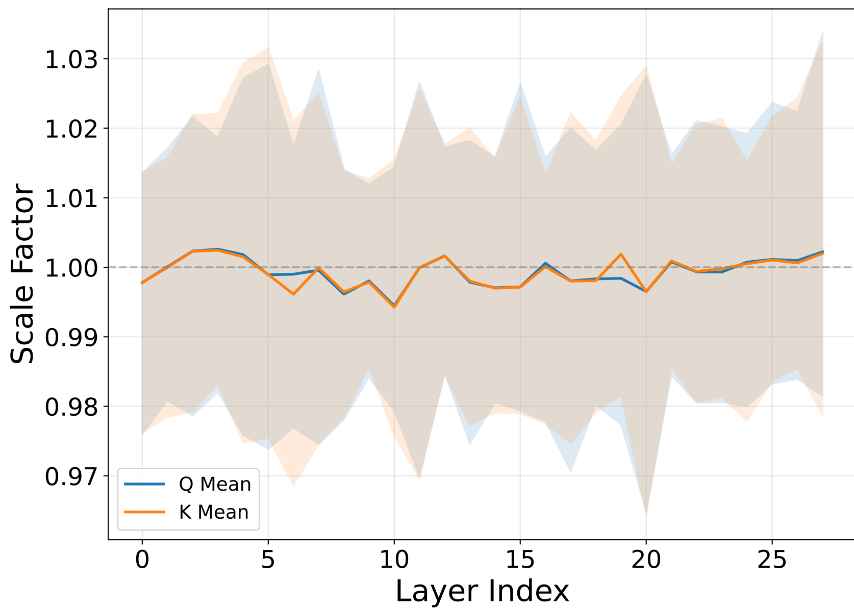
(d) Llama Math ( \alpha=0.3 )
