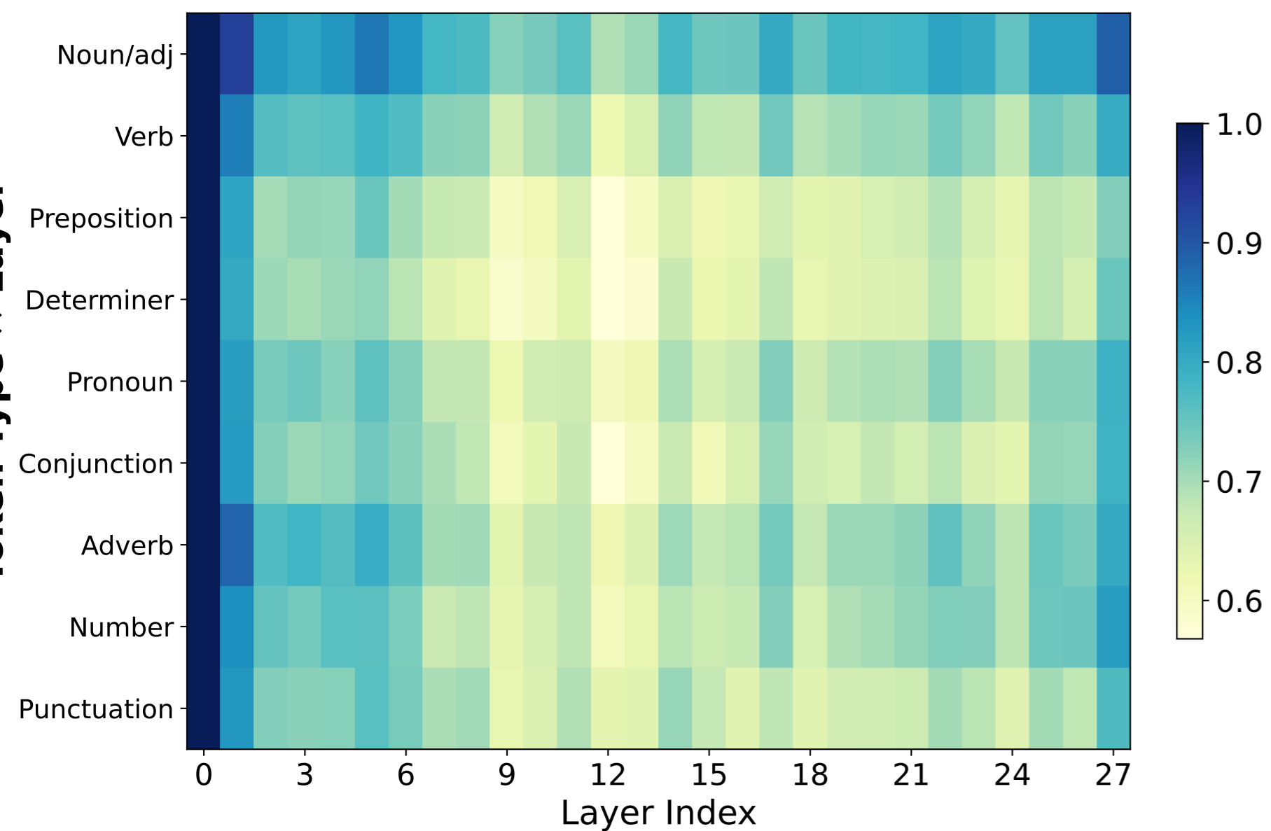
Llama-3.2-3B (RoPE)
